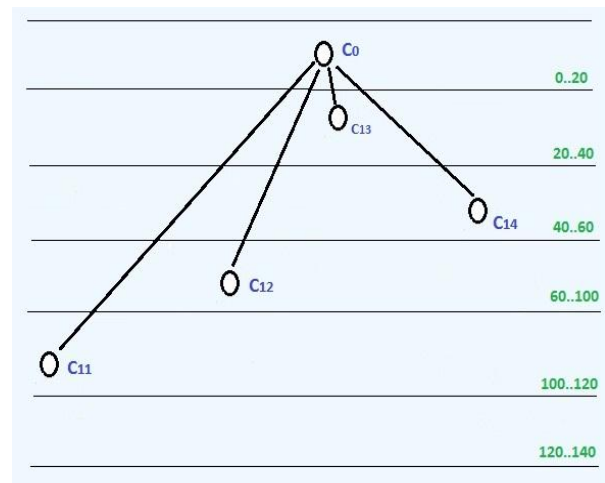
Рисунок 4 – Позиція входження посилання на інше поняття в статті Wikipedia
