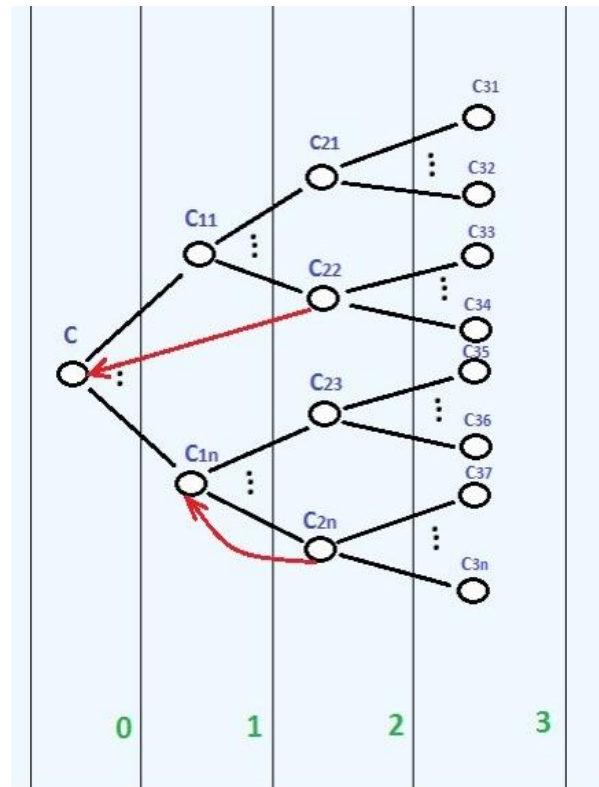
Рисунок 2 – Приклад набору понять, коли поняття другого рівня вкладеності посилаються на поняття першого або нульового рівня вкладеності.
