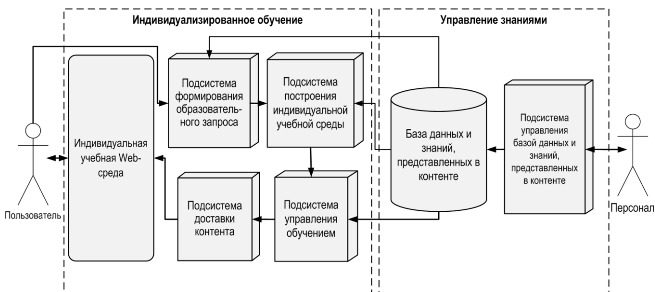
Рис.1. Концептуальная схема программной системы управления контентом ИУП
